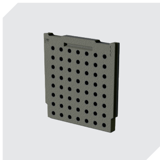
Isolierbox-Querteiler L 298 x B 25 x H 294 mm 79-51050
