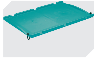
Auflagedeckel einseitig anschnürt montiert auf Kleinladungsträger KLT L 600 x B 400 mm 43-21523
