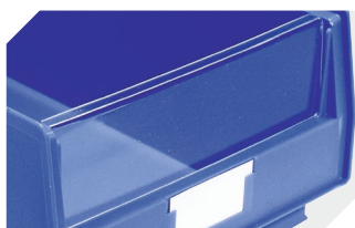
Visière pour bacs à bec, série PK l 277,5 x l 14,5 x H 81 mm 2-1114
