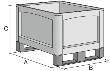
Pos. Abmessungen, Toleranzen nach DIN 16901
