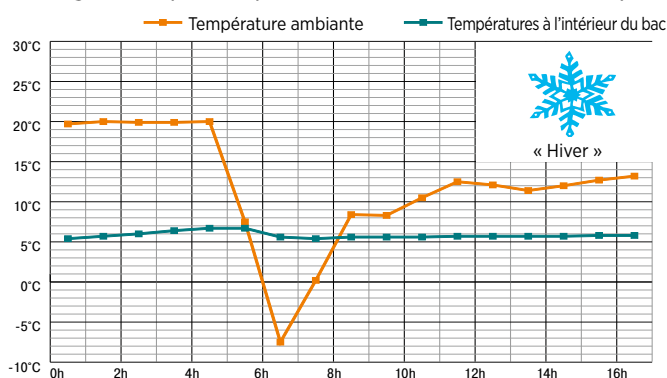
« Hiver » Ligne temps-température avec isolation thermique
