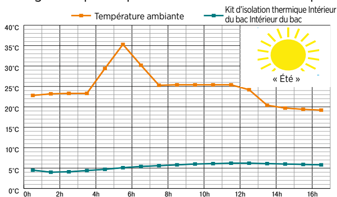
« Été » Ligne temps-température avec isolation thermique
