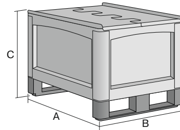
Pos. Abmessungen, Toleranzen nach DIN 16901
